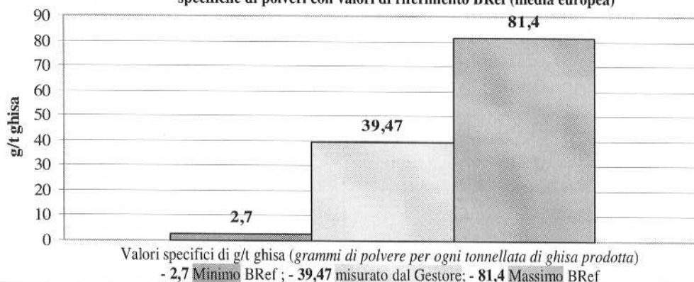
Figura 13 - Fase di processo Caricamento materiali - Comparazione delle emissioni specifiche di polveri con valori di riferimento BRef (media europea)
