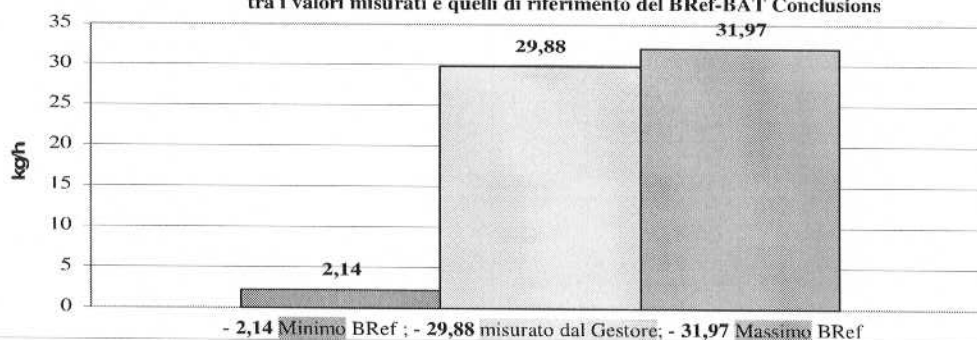
Figura 14 - Fase di processo Caricamento - Differenza in massa delle polveri emesse tra i valori misurati e quelli di riferimento del BRef-BAT Conclusions
