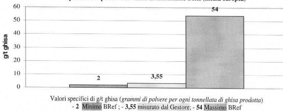
Figura 15 - Fase di processo P.C.I. - Comparazione delle emissioni specifiche di polveri con valori di riferimento BRef (media europea)
